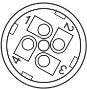
Цоколевка соединителя (вид со стороны монтажа)
