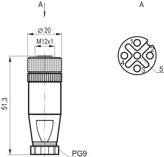
Габаритный чертеж
