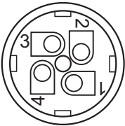
Цоколевка соединителя (вид со стороны монтажа)
