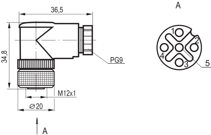
Габаритный чертеж
