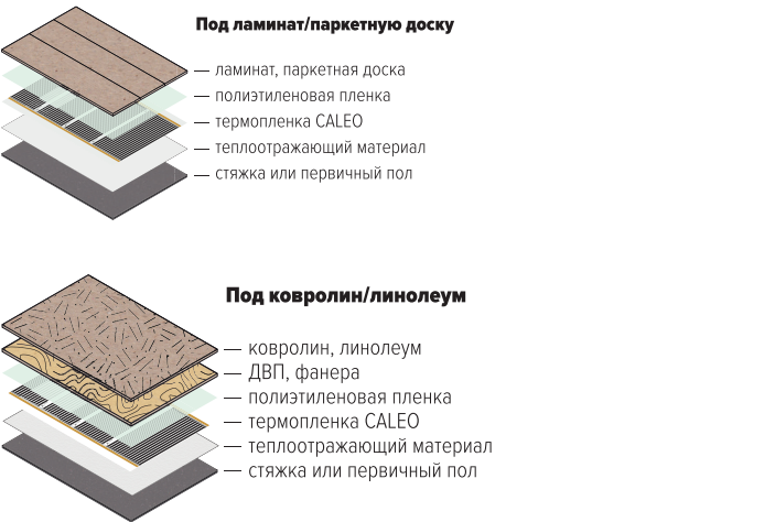
Рис. Схема монтажа теплого пола CALEO под ламинат, ковролин, линолеум
