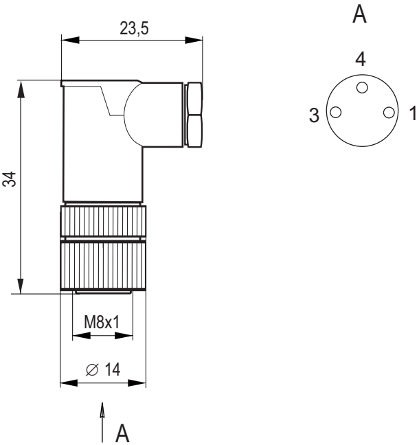
Габаритный чертеж
