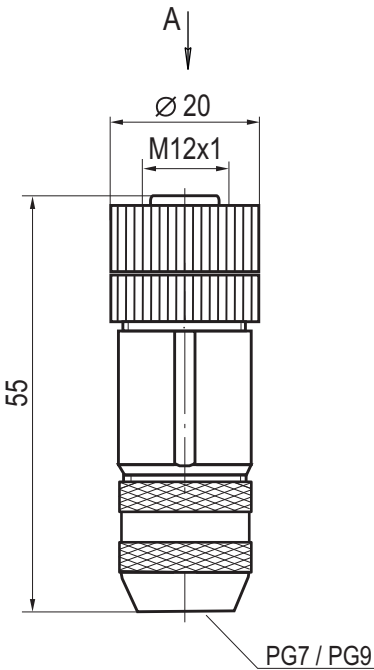
Габаритный чертеж
