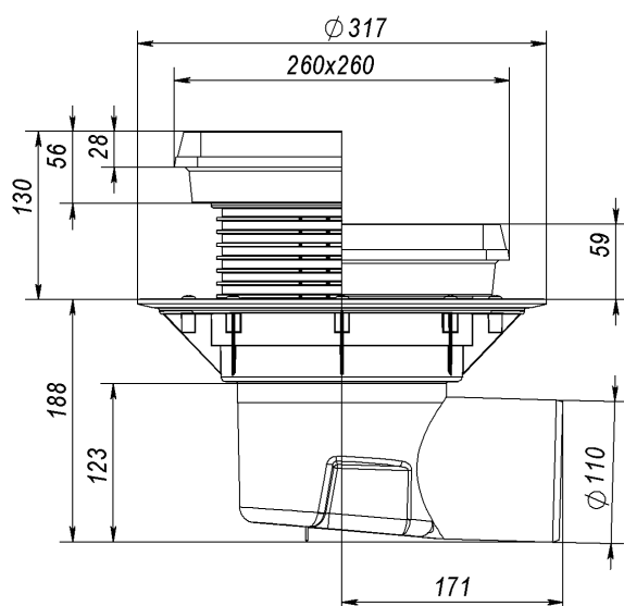
Рис.2 Чертеж трапа серии 615
