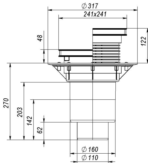
Рис.3 Чертеж трапа серии 616
