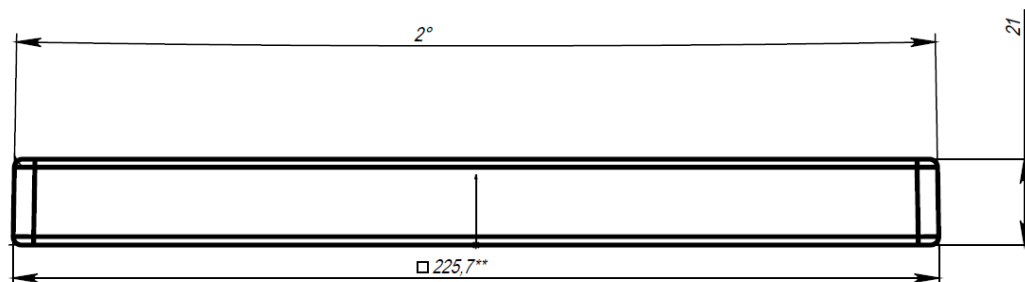
Рис. 1 Чертеж чугунной решетки
