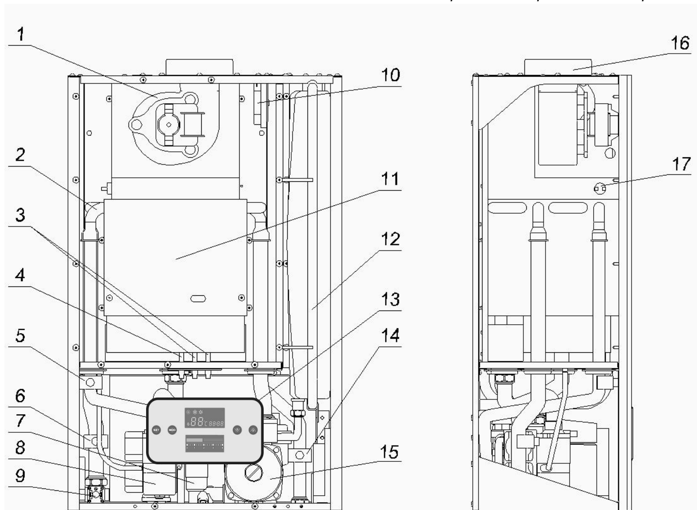
Рис. 3 Функциональная схема котла серии Amulet Turbo SB
