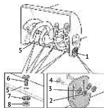
1 – ограничительная лыжа; 2, 8 – гайки; 3, 7 – шайбы; 4, 6 – болты; 5 – струг.
