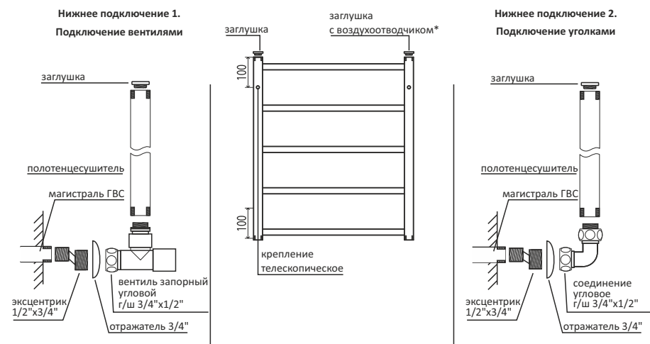
Схема 1. Нижнее подключение
