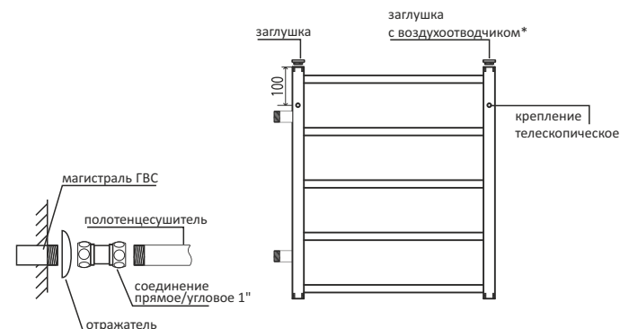
Схема 2. Боковое подключение
