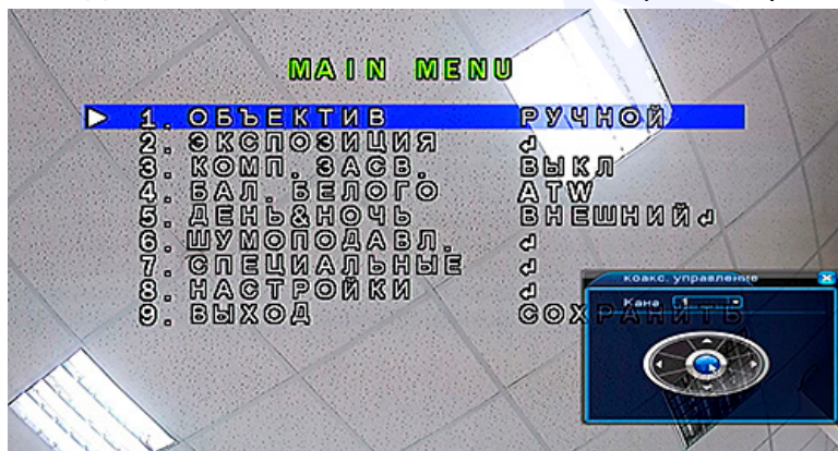
Рис. 3.16 Управление по коаксиалу
