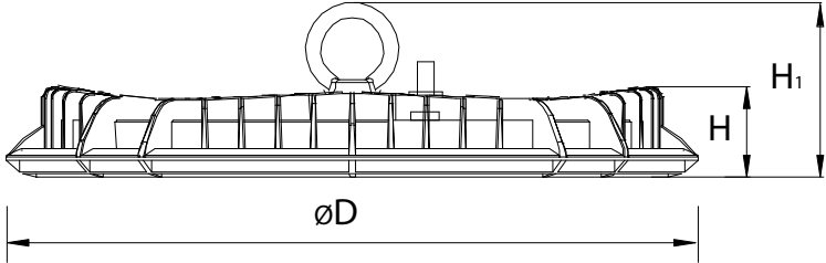
Рис. 1 Светильник РНВ UFO 04
