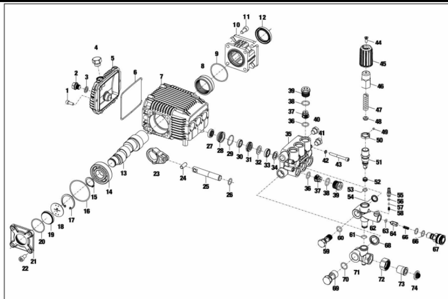
Лист деталей
