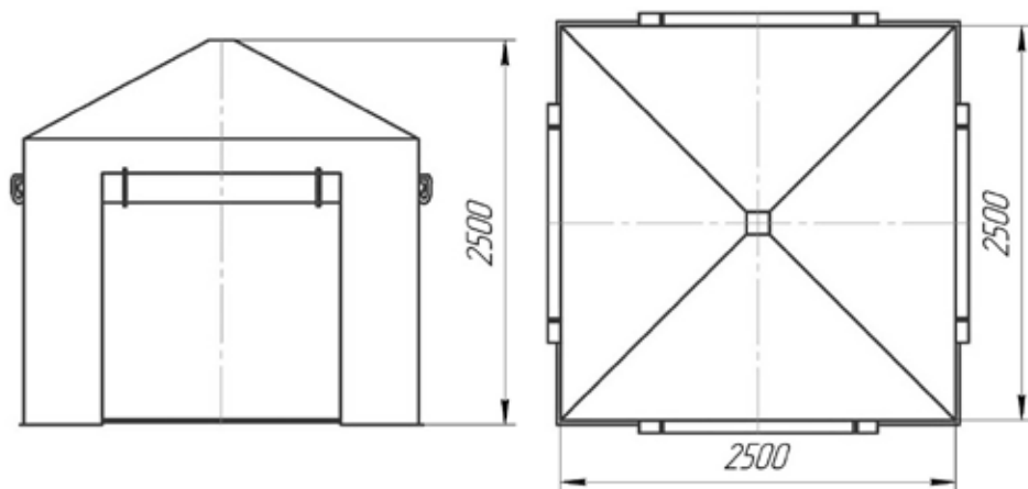
Рис. 1. Общий вид палатки сварщика.
