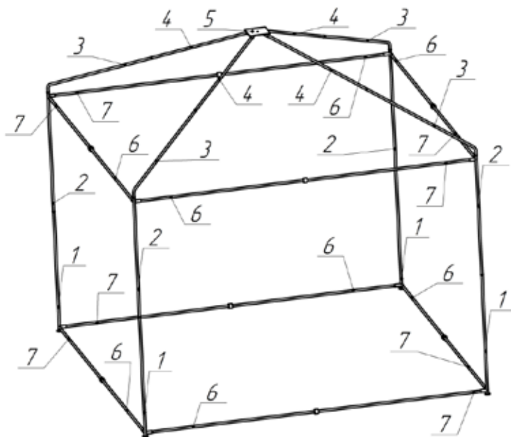
Рис. 2. Общий вид каркаса палатки сварщика.
