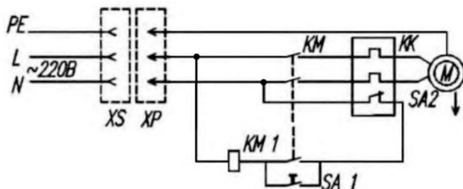
Рис. 2 Схема электрическая принципиальная
