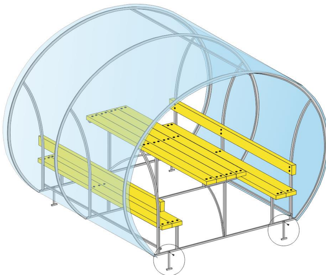
Рис. 6 Общий вид крепления основания беседки к земле.
