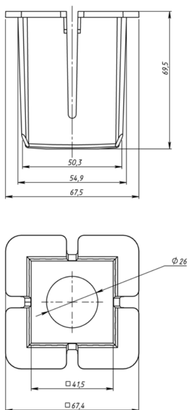
Рис. 3. Размеры вставки опоры EASY FOOT 41
