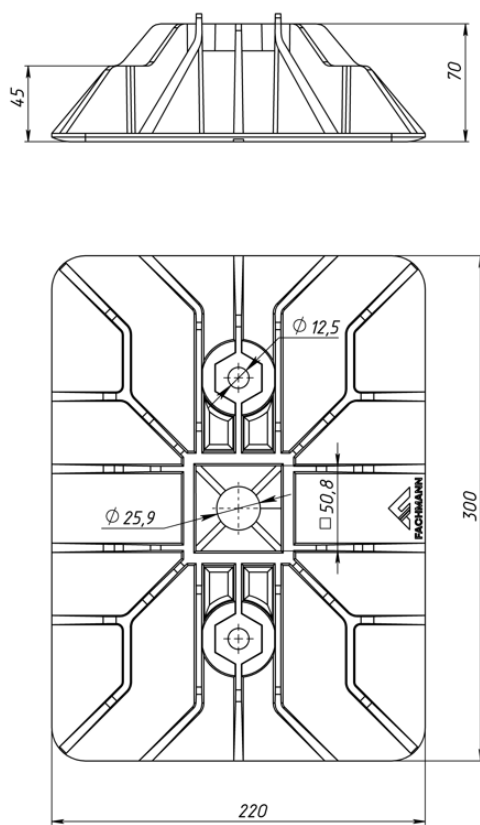
Рис. 2. Размеры кровельной опоры EASY FOOT 300x220 41/21
