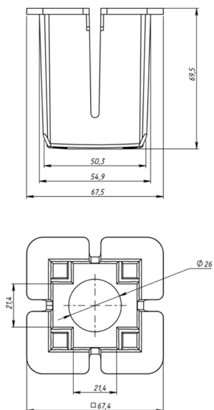
Рис. 4. Размеры вставки опоры EASY FOOT 21
