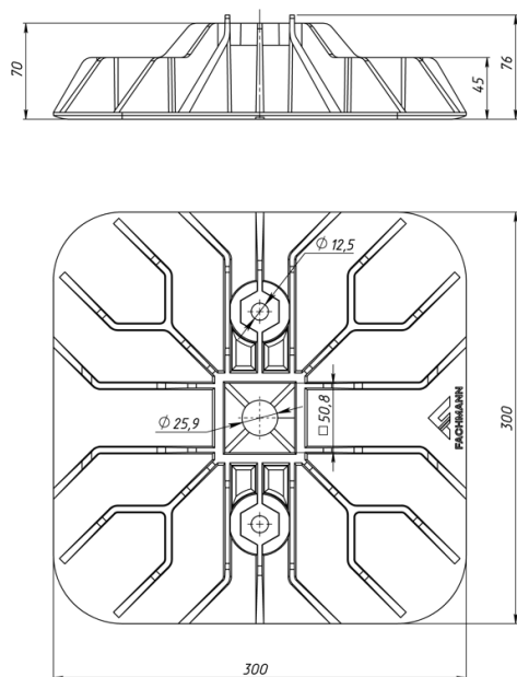
Рис. 1. Размеры кровельной опоры EASY FOOT 300x300 41/21
