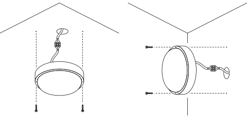
Рис. 2. Пример монтажа
