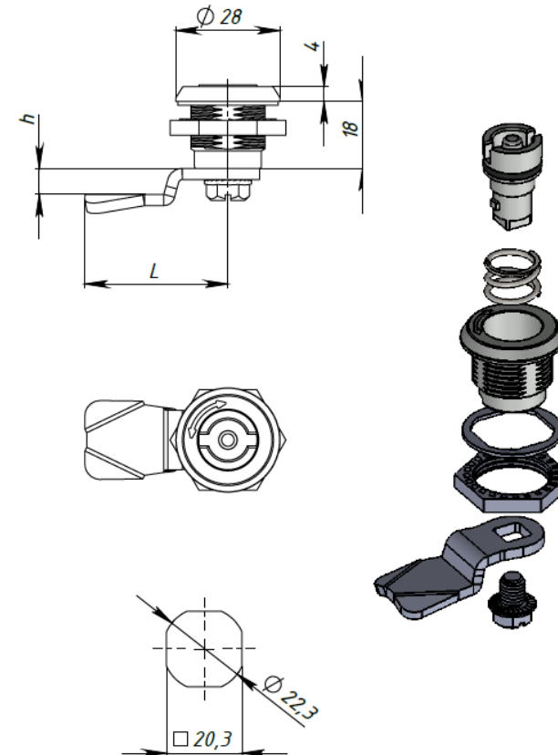
Чертеж замка под ключ две бородки
