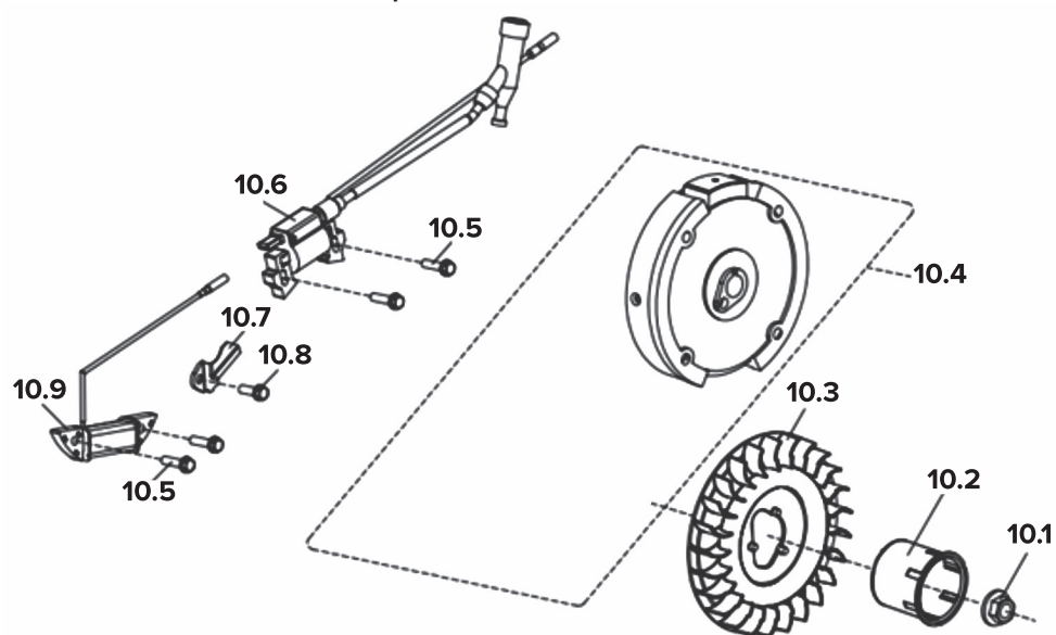
Схема сборки № 10
