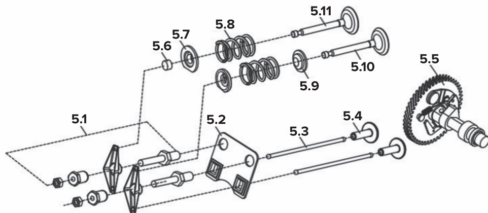
Схема сборки № 5
