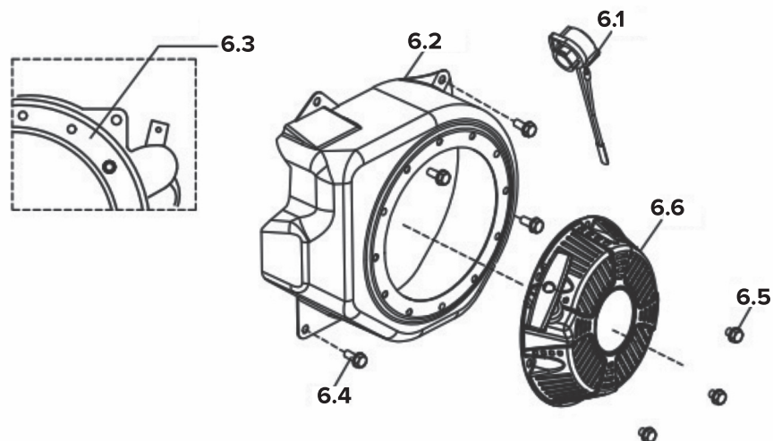
Схема сборки № 6
