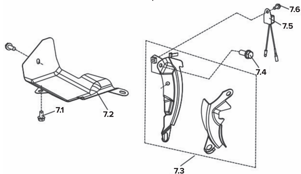
Схема сборки № 7
