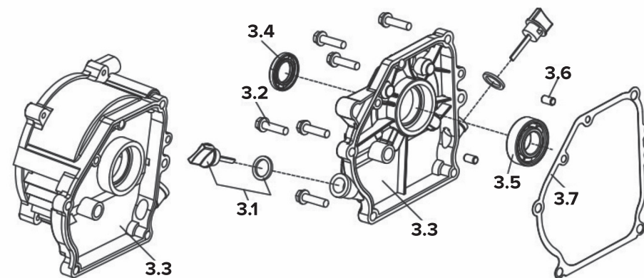
Схема сборки № 3
