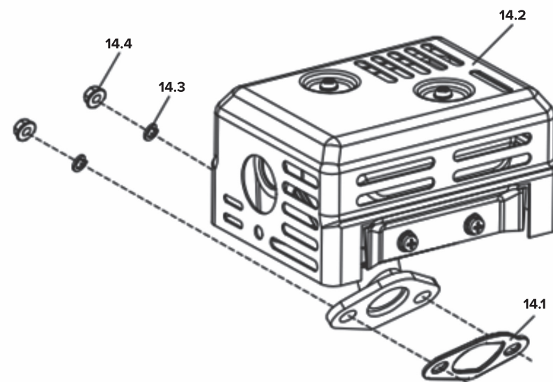
Схема сборки № 14
