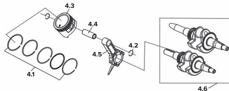
Схема сборки № 4
