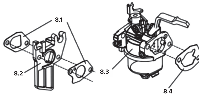
Схема сборки № 8
