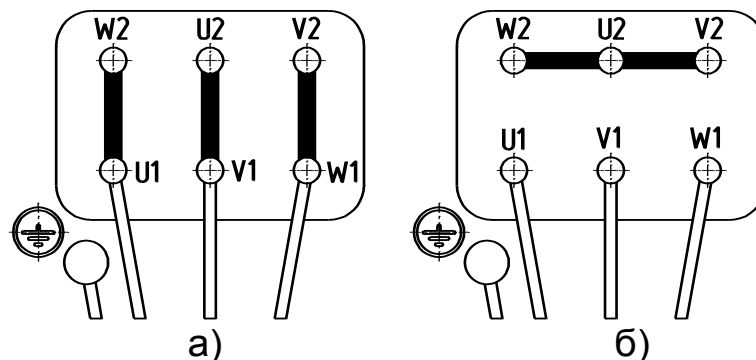
Рисунок 2. Схема соединения обмоток статора: а) в треугольник – напряжение 220 В; б) в звезду – напряжение 380 В.
