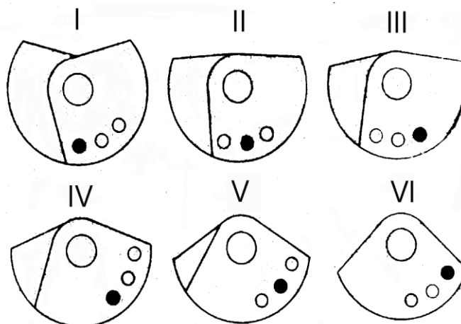
Рисунок 5. Схема регулировки статического момента ИВ – 104Б, ИВ-104Н, ИВ-104Б-6, ИВ-104Н-6, ИВ-106Э, ИВ-106Э1, ИВ – 127, ИВ-127Н, ИВ-127Э
