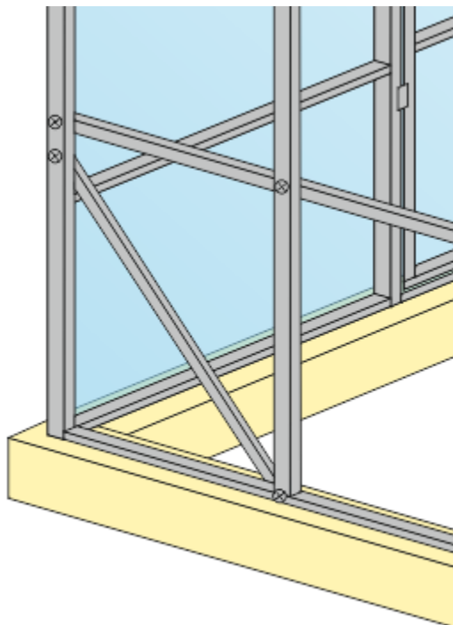
Рис. 14 Установка раскосов
