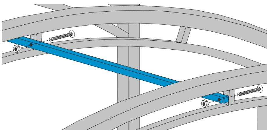
Рис № 13. Установка стяжек на крыше
