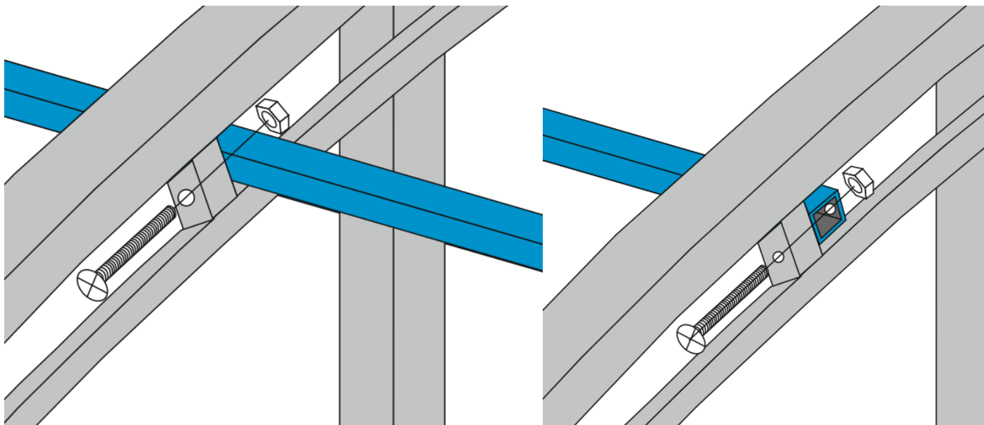
Рис № 12. Установка стяжек на крыше
