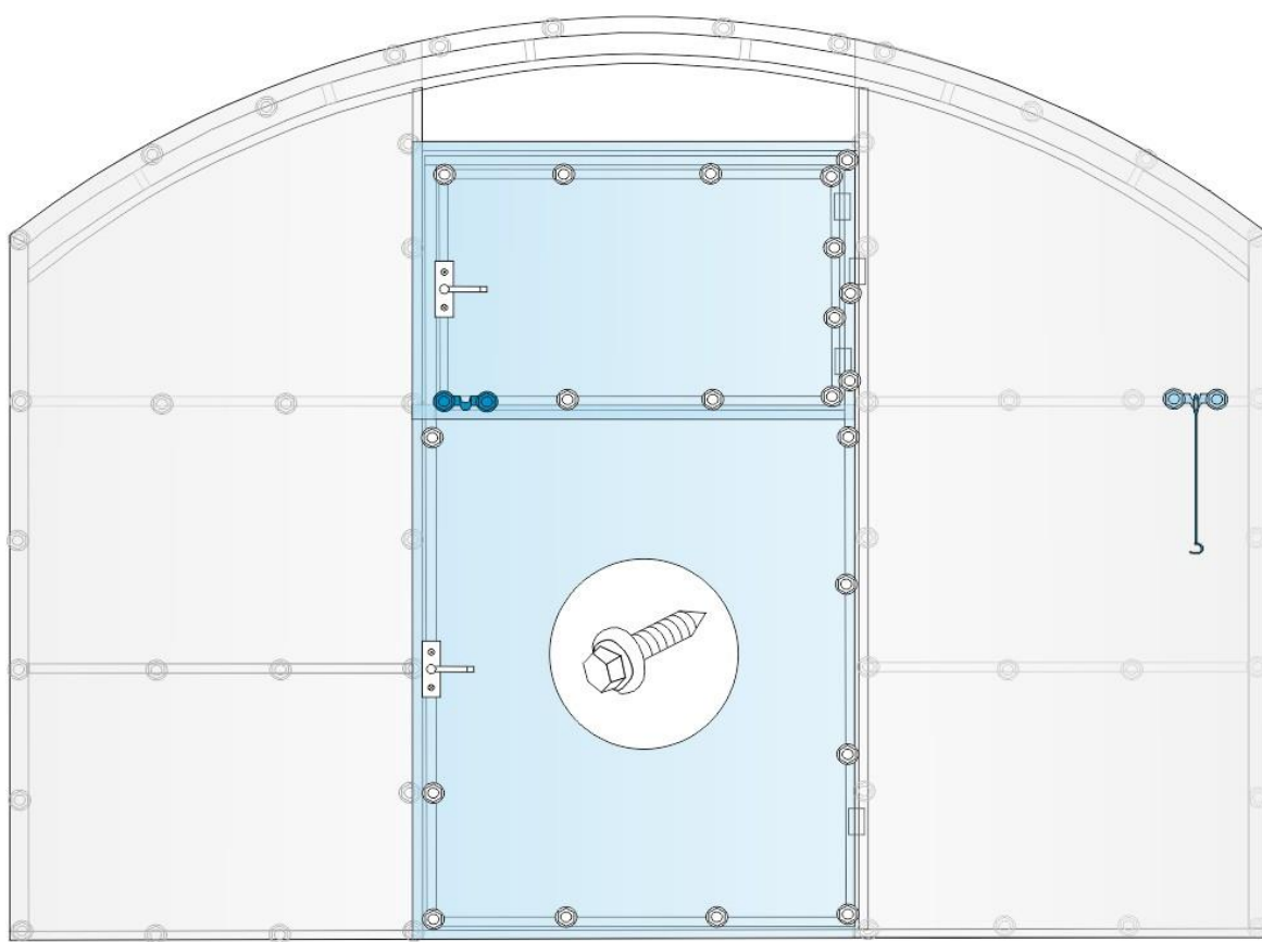
Рис № 3. Точки крепления саморезов на торцах теплицы.
