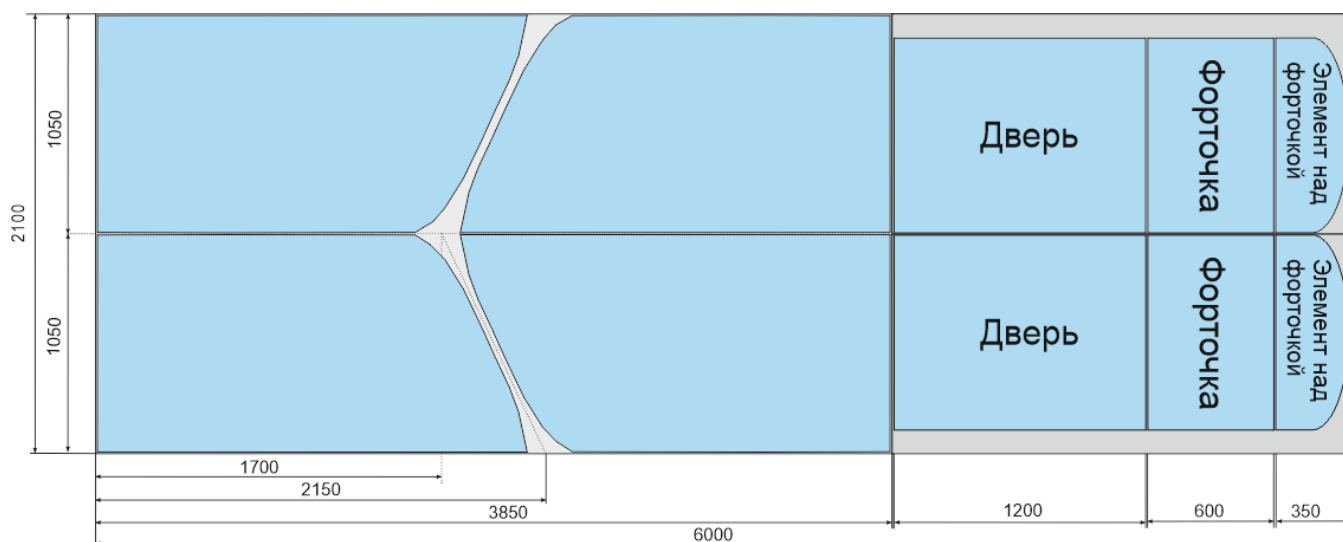
Рис № 2. Схема раскроя поликарбоната на торцевые части теплицы.
