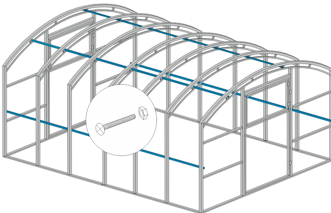
Рис № 11. Соединение торцов и дуг
