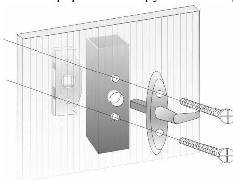
Рис № 5 а. Установка ручки.
