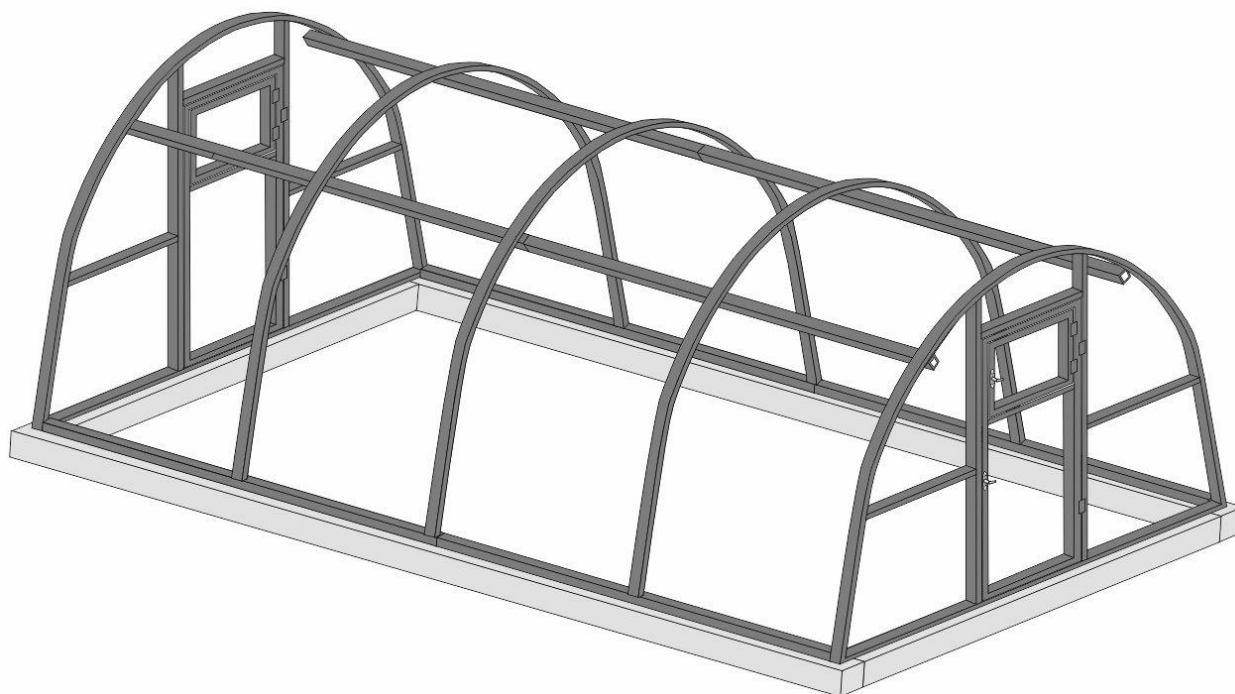
Рис № 11. Установка дуг.
