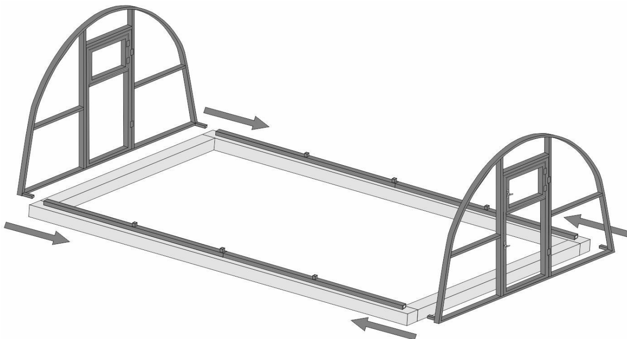
Рис № 10. Установка торцов.
