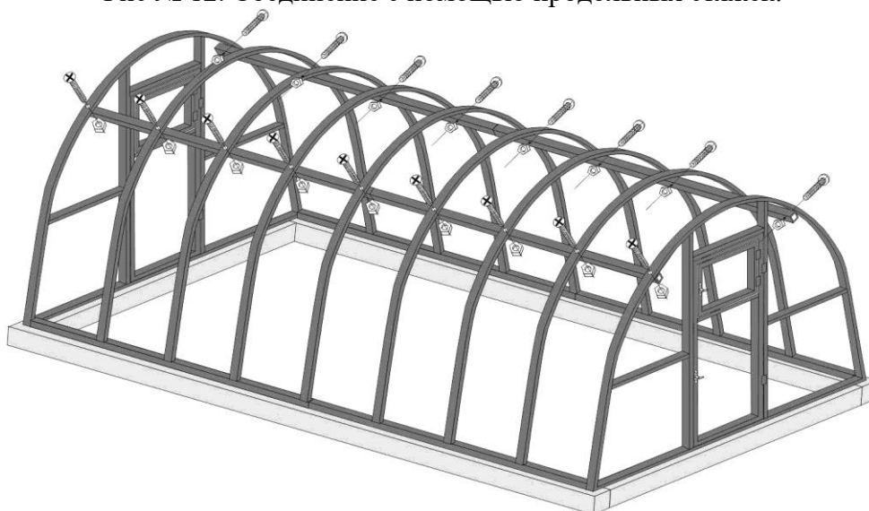
Рис № 13. Общий вид соединительных узлов.
