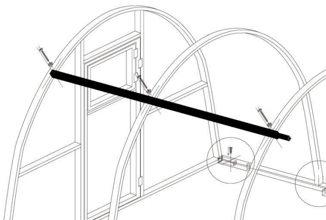
Рис № 12. Соединение с помощью продольных стяжек.
