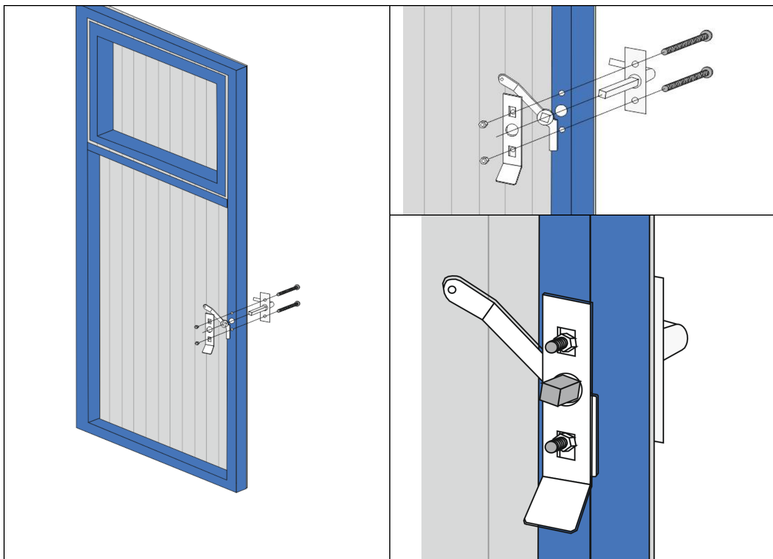
Рис № 6. Установка ручки и замка с фиксатором на двери.
