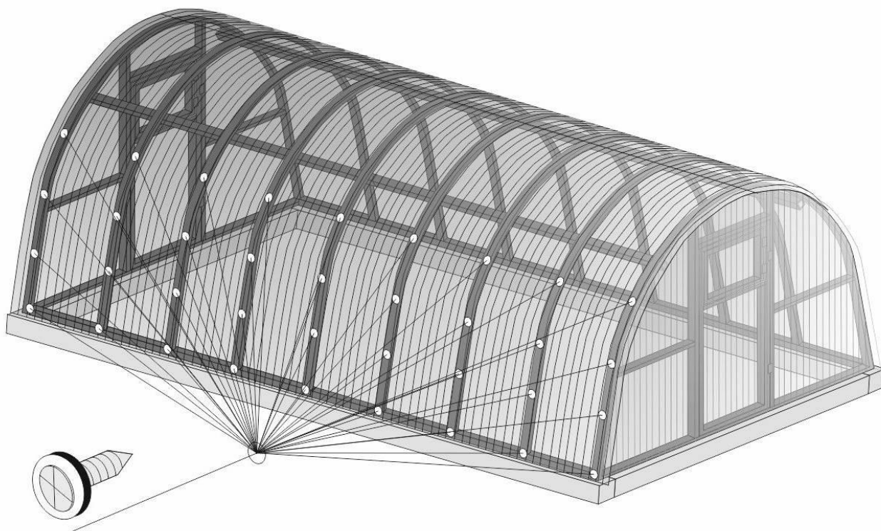
Рис № 14. Точки крепления саморезов на верхней части теплицы.
