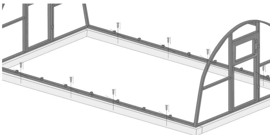
Рис № 12. Крепление к фундаменту.
