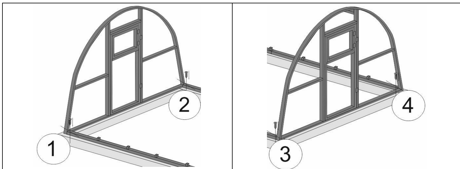
Рис № 11. Места стыковки соединяем саморезами (позиции № 1, 2, 3, 4).
