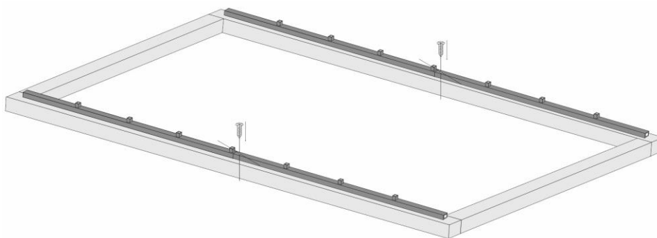
Рис № 8. Соединение продольных элементов.
