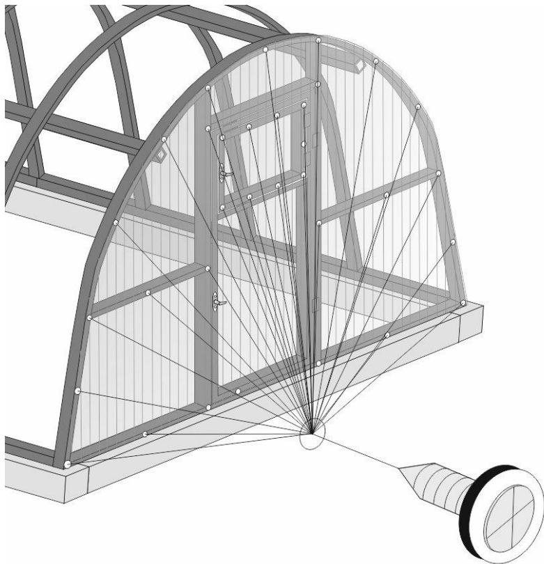
Рис № 3. Точки крепления саморезов на торцах теплицы.
