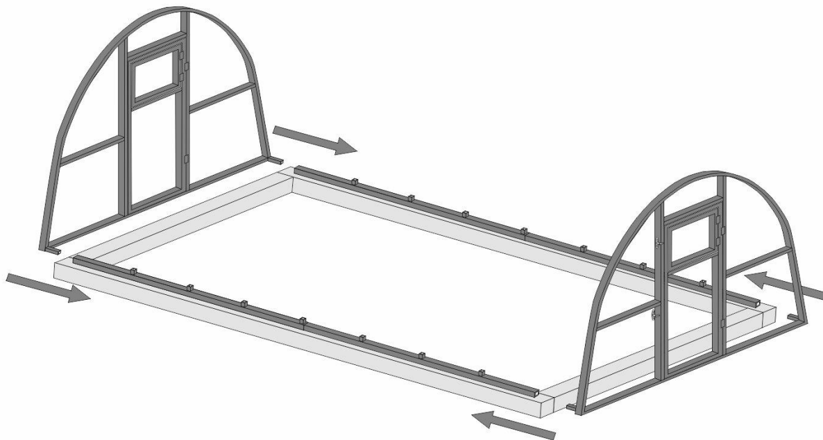
Рис № 10. Установка торцов.
