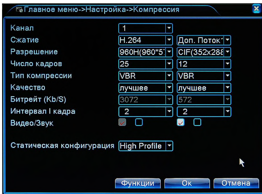
Рис. 4.3.2. Настройка. Сжатие
