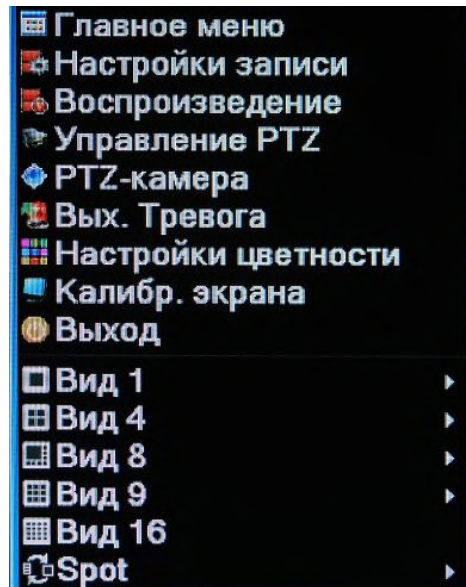
Рис. 3.1. Всплывающее меню
