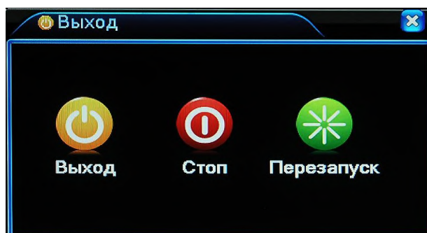
Рис. 4.4.9. Управление. Выход
