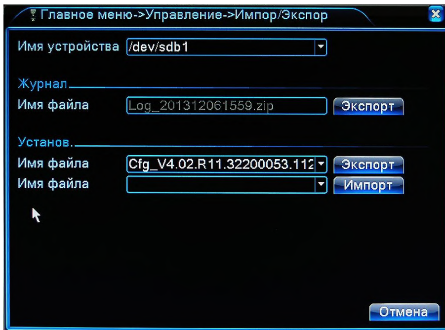
Рис. 4.4.8. Управление. Импорт/экспорт
