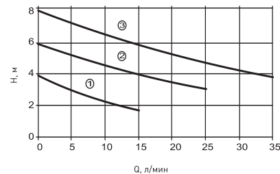
Рабочее поле для насосов С-25/8
