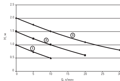
Рабочее поле для насосов С-25/4, С-25/4-130 и С-32/4
