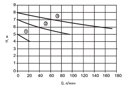
Рабочее поле для насосов С-32/8
