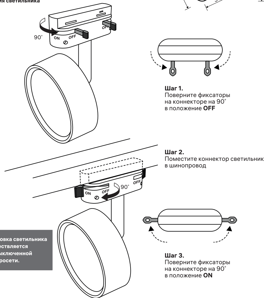
Схема подключения светильника
