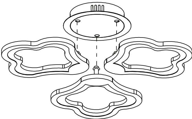
2. Схема крепления плафона к основанию
