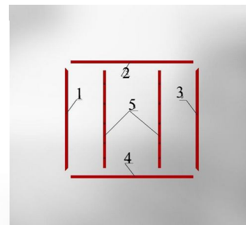
Рис. 2 Схема сборки щита пожарного открытого каркасного разборного
