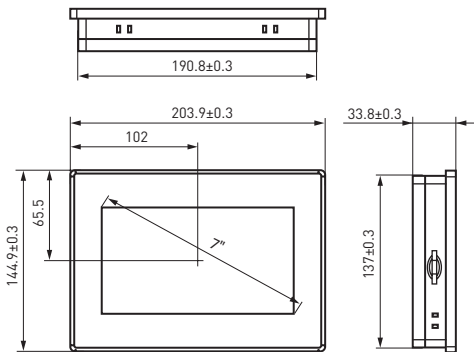
Рис. 2 – Габаритные размеры RSC-7 и RSC-7E
