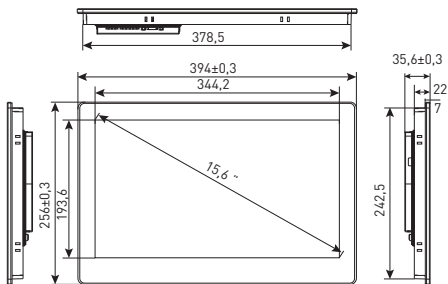
Рис. 4а – Габаритные размеры RSC-15E
