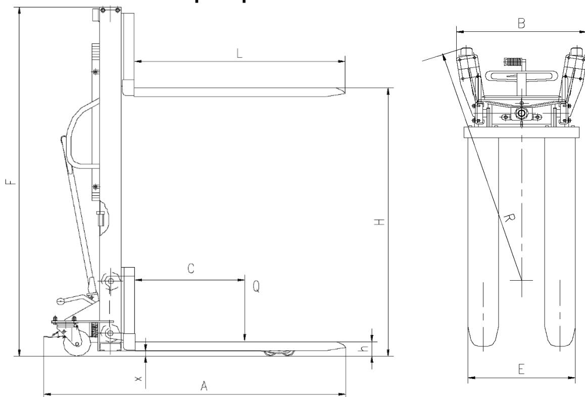
Рис.1 - Габаритные размеры штабелера ручного СТУ-ЕН
