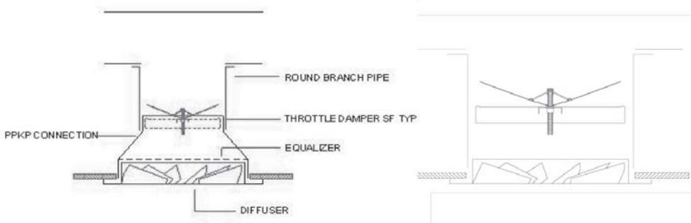
Установка в стальной канал
