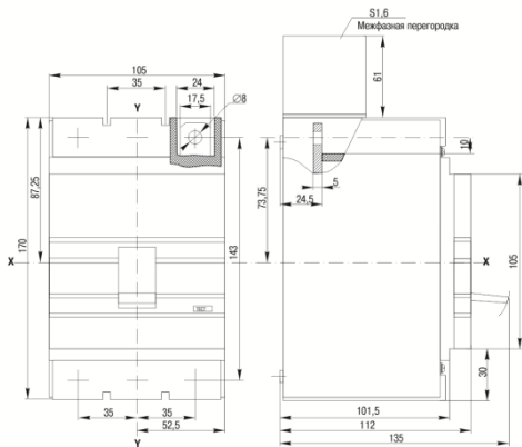
Рисунок 7 - Габаритные и установочные размеры выключателя ВА88-35
