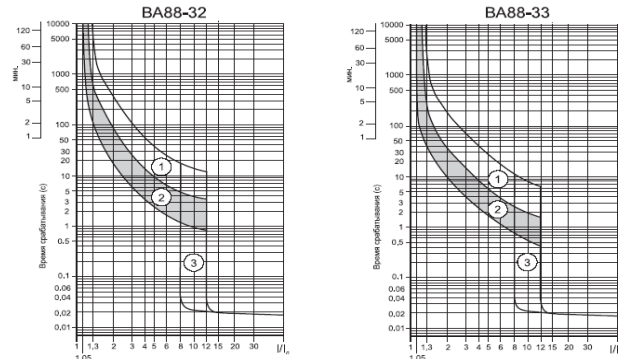
Рисунок 1. Время-токовые характеристики выключателей ВА88-32 и ВА-33 в условиях одновременной нагрузки всех фазных полюсов.
