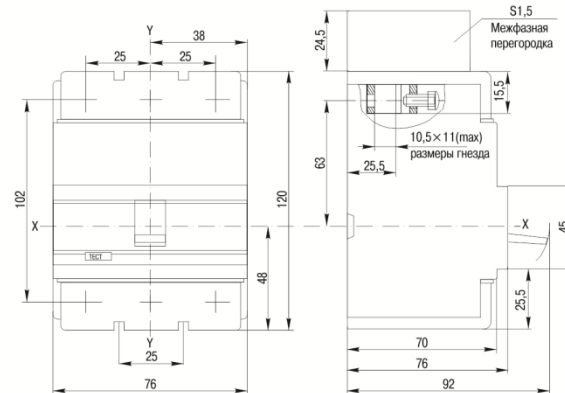
Рисунок 5 - Габаритные и установочные размеры выключателя ВА88-32
