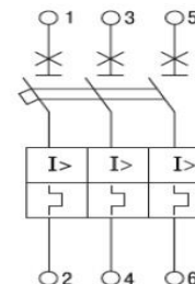
Рисунок 4 — Электрическая схема выключателя с тепловым и электромагнитным расцепителем.
