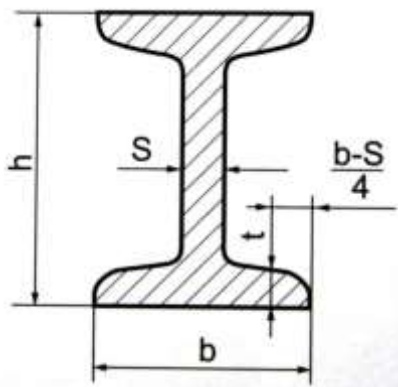
Рисунок 5. Двутавровая балка.
