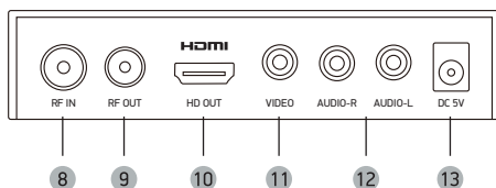
Общий вид задней панели
