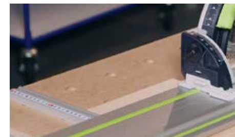
Подвижной упор КТ МV свободно перемещается в верхнем пазу профиля-упора КТ ЕМ
