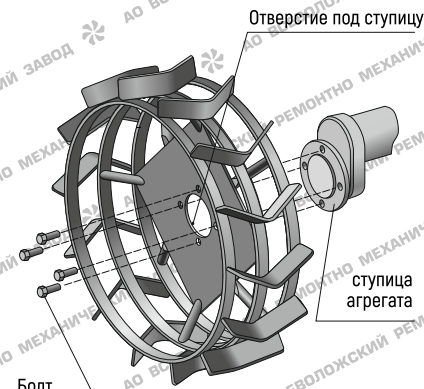
③ Установка на ступицу агрегата
