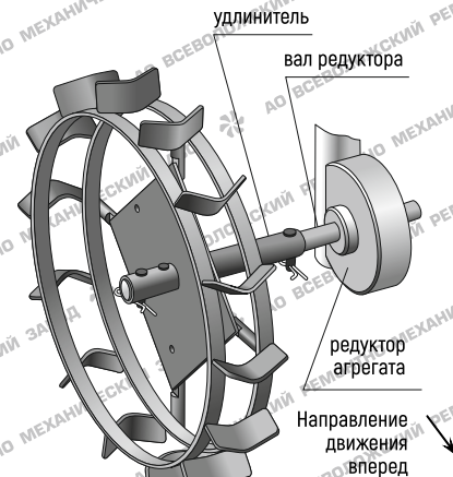
② Установка на вал редуктора через удлинитель (для увеличения колеи)
