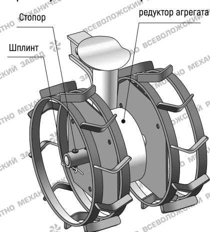
① Установка на вал редуктора
