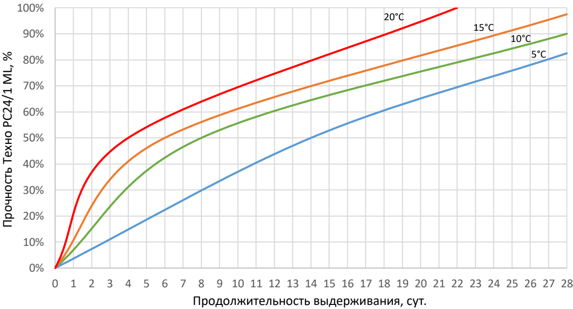
Рис.1. Прочность цементной штукатурки Техно PC24/1 ML в зависимости от температуры и продолжительности выдерживания.
