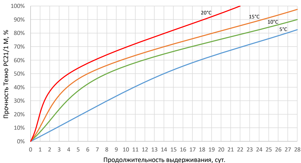
Рис.1. Прочность цементной штукатурки Техно РС21/1 М в зависимости от температуры и продолжительности выдерживания.
