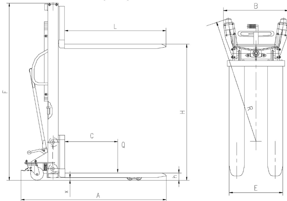
Рис.1 - Габаритные размеры
