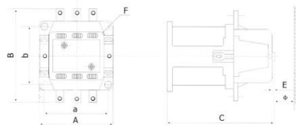
Рисунок 3 - Габаритные и присоединительные размеры пускателей 40-95А
