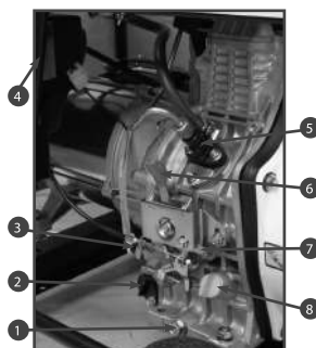
Рис. 3 Двигатель, вид со стороны панели управления
