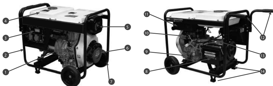
Рис. 1 Основные узлы и органы управления
