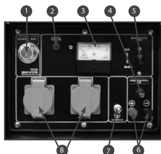
Рис.2 Панель управления
