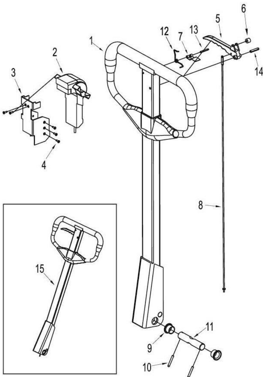
Схема 1. Ручка в сборе.
