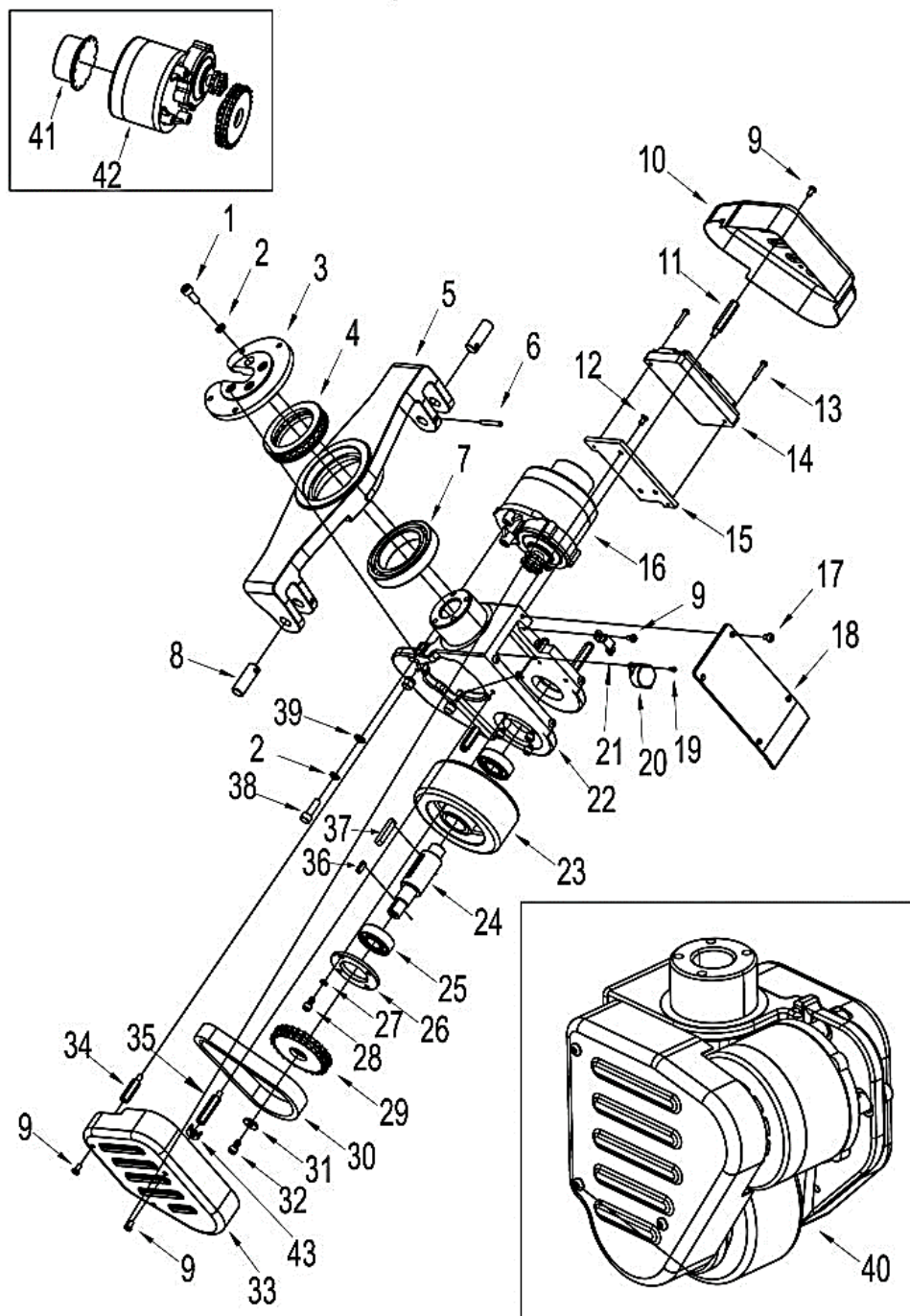
Схема 2. Привод.
