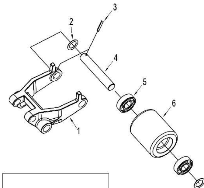
Схема 6. Колеса.
