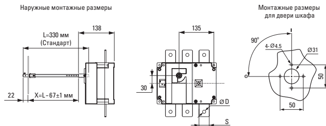
Рисунок 12г – Монтажные размеры при установке на дверцу шкафа для рубильников 400-630 А
