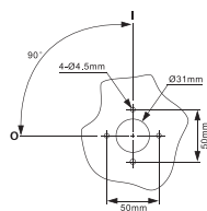
Монтажные размеры для двери шкафа
