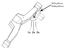
Рисунок 11б – Блокировка ручки рубильников 2000-3150 А навесным замком
