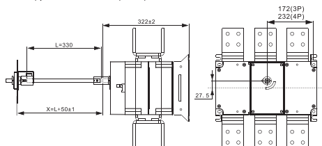
Наружные монтажные размеры
