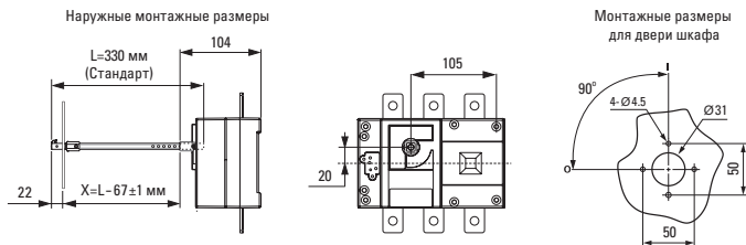
Рисунок 12в – Монтажные размеры при установке на дверцу шкафа для рубильников 250 А
