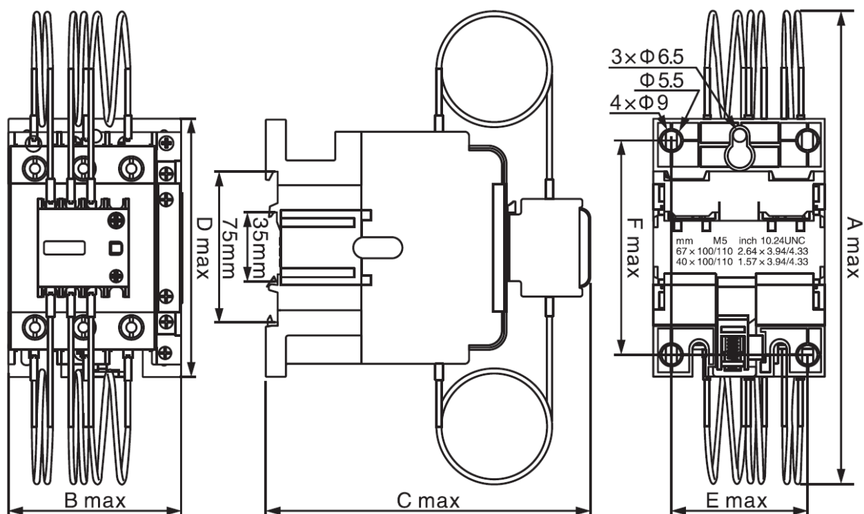
Габаритные и установочные размеры КМ-102-CAP 30 ~ 60 кВар.
