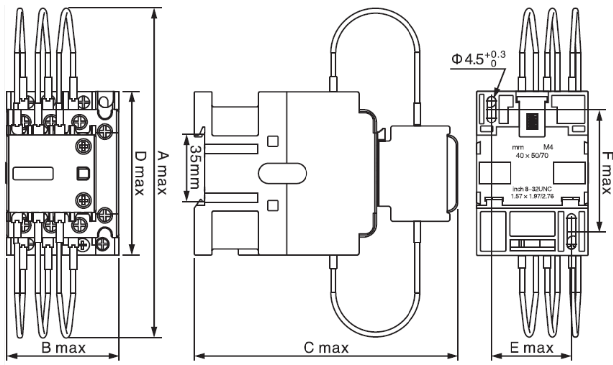
Габаритные и установочные размеры КМ-102-CAP 12 ~ 25 кВар.
