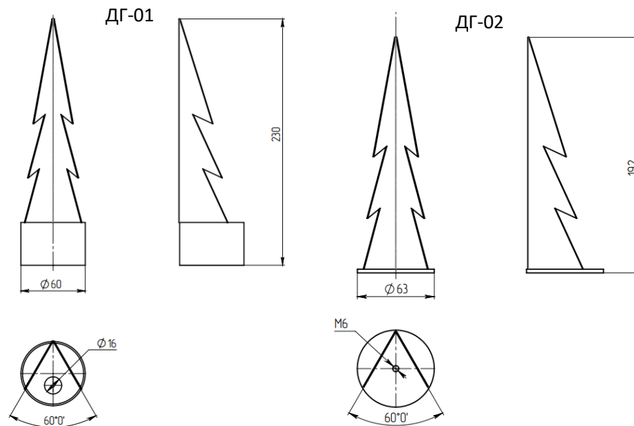
Рисунок 1. Общий вид держателей ДГ-01 и ДГ-02
