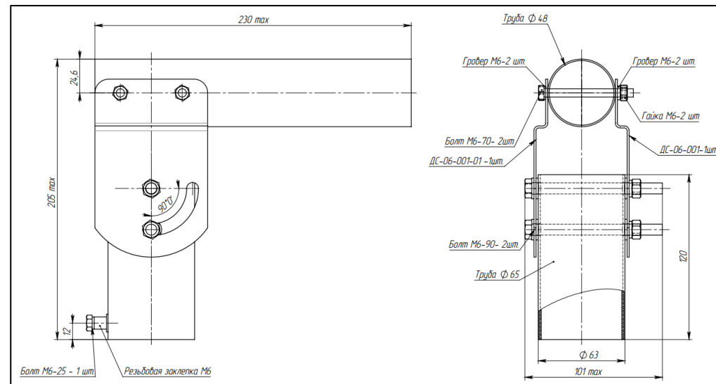
Рисунок 1. Сборочный чертёж ДС-06
