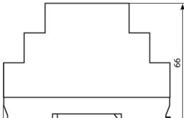
Рис2. Размеры корпуса.
