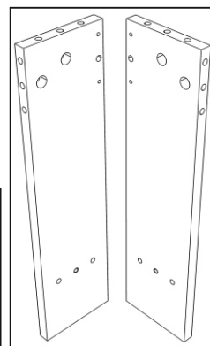
8. Стойка (2 лев. и 2 прав.)
